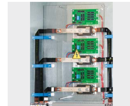
Тиристорные коммутаторы
